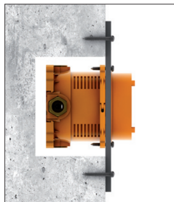
In-wall installation Inwand-Montage Montage dans le mur Montaggio in parete
