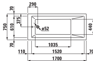
23195.1 ** Bathtub, with frame, sanitary acrylic, 1700x750 mm Badewanne, mit Fussgestell, Sanitäracryl, 1700x750 mm Baignoire, avec piétement, acrylique sanitaire, 1700x750 mm Vasca, con base, in acrilico sanitario, 1700x750 mm
