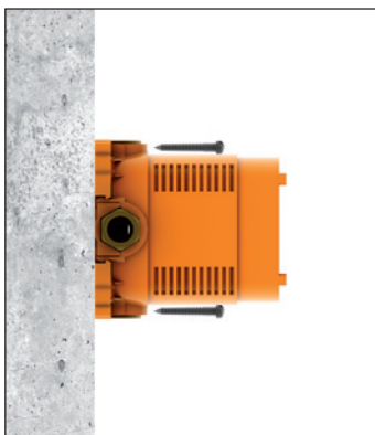
On-wall installation Vorwand-Montage Montage sur le mur Montaggio davanti alla parete
