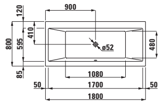
23295.1 ** Bathtub, with frame, sanitary acrylic, 1800x800 mm Badewanne, mit Fussgestell, Sanitäracryl, 1800x800 mm Baignoire, avec piétement, acrylique sanitaire, 1800x800 mm Vasca, con base, in acrilico sanitario, 1800x800 mm
