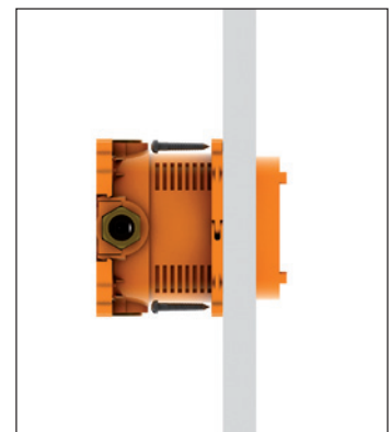
Behind-wall installation Hinterwand-Montage Montage derrière le mur Montaggio dietro alla parete
