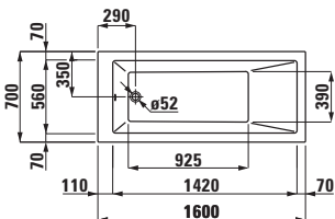
23395.1 ** Bathtub, with frame, sanitary acrylic, 1600x700 mm Badewanne, mit Fussgestell, Sanitäracryl, 1600x700 mm Baignoire, avec piétement, acrylique sanitaire, 1600x700 mm Vasca, con base, in acrilico sanitario, 1600x700 mm
