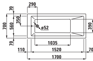
23095.1 ** Bathtub, with frame, sanitary acrylic, 1700x700 mm Badewanne, mit Fussgestell, Sanitäracryl, 1700x700 mm Baignoire, avec piétement, acrylique sanitaire, 1700x700 mm Vasca, con base, in acrilico sanitario, 1700x700 mm
