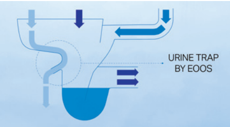
URINABTRENNUNG
