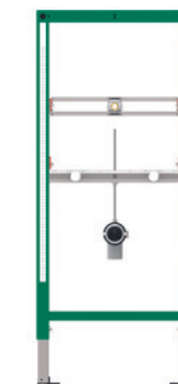
Waschtisch-Elemente
