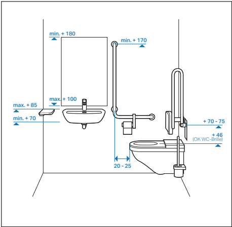
Öffentliches WC
