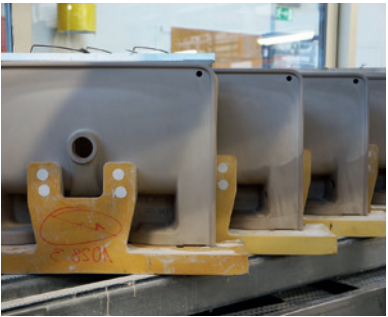
SAPHIRKERAMIK IN DER PRODUKTION MIT DER VON LAUFEN ENTWICKELTEN DRUCKGUSSTECHNIK
