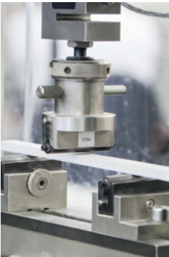
SAPHIRKERAMIK VERFÜGT ÜBER EINE BIS ZWEIFACH STÄRKERE BIEGEFESTIGKEIT
